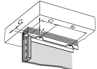
Fijación de carril de cabezal de desvío con placas de yeso (opcional con sellador)
