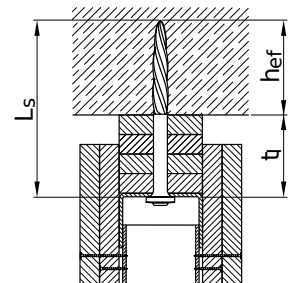
Umlenkkopfbefestigung mit Gipsstreifen (optional mit Dichtmasse)
