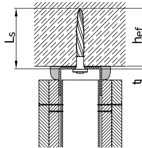
Profilbefestigung Umlenkopf (optional mit Dichtmasse)
